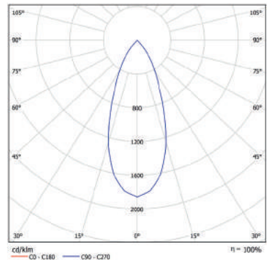
ANTLIA LED1X2300 D343 T840
